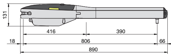
MÉRETEK
