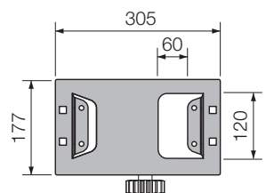
RÖGZÍTŐ ALAP ALKATRÉSZSZÁM RPIAFEVOZ
