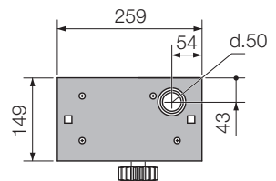
RÖGZÍTŐ ALAP ALKATRÉSZ SZÁM PIAFACE300AS
